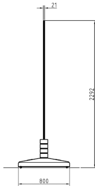
Seite
